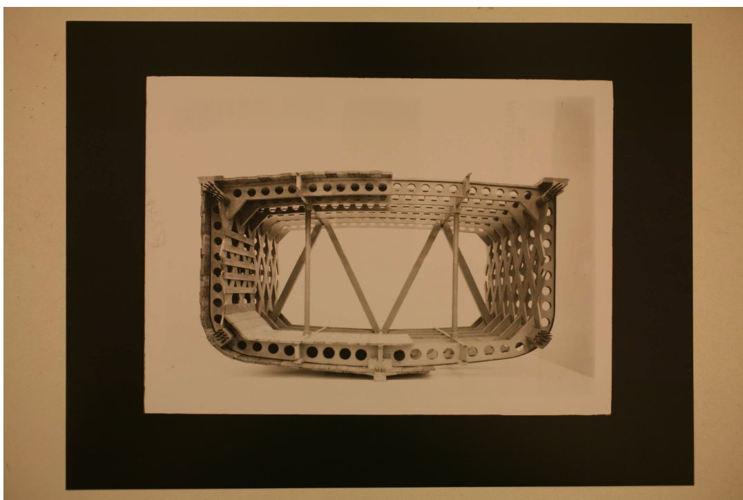
Fig. 109, Archivio Vasari, (Motoveliero ad elementi prefabbricati), 1942-43, CSAC, sezione fotografia.
