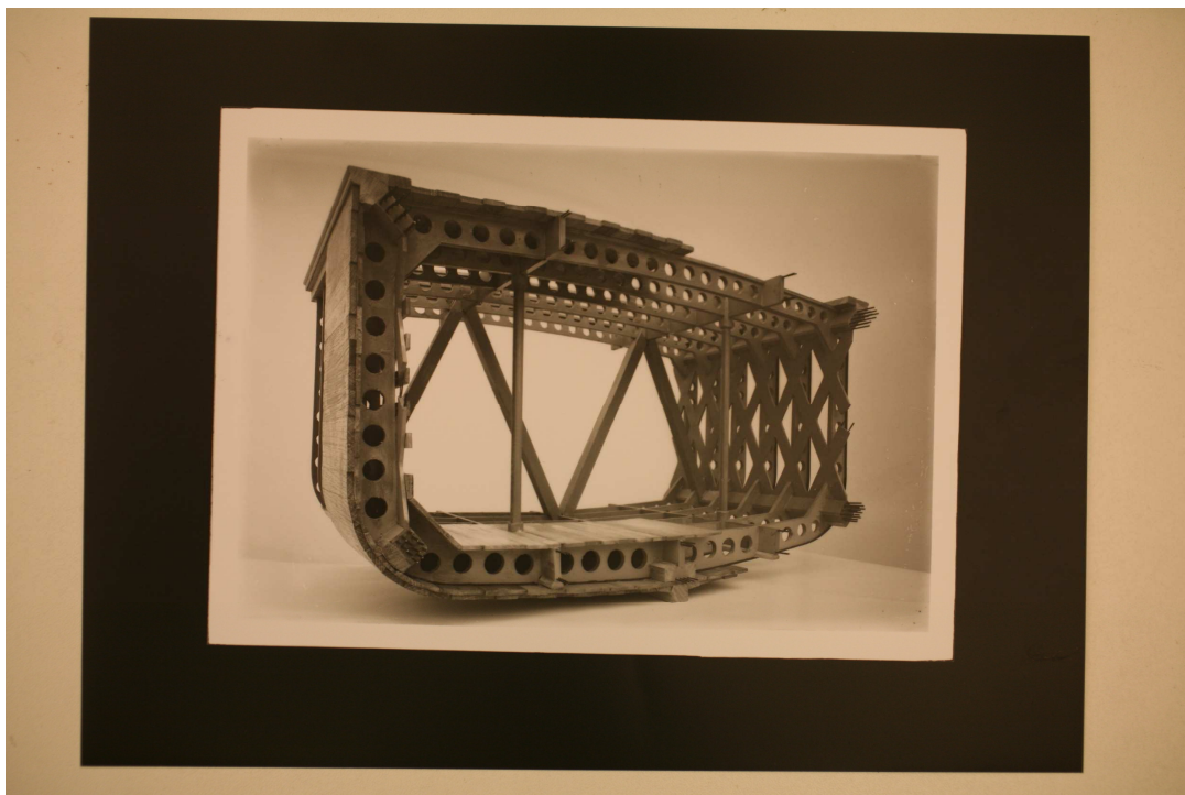
Fig. 108, Archivio Vasari, (Motoveliero ad elementi prefabbricati), 1942-43, CSAC, sezione fotografia.
