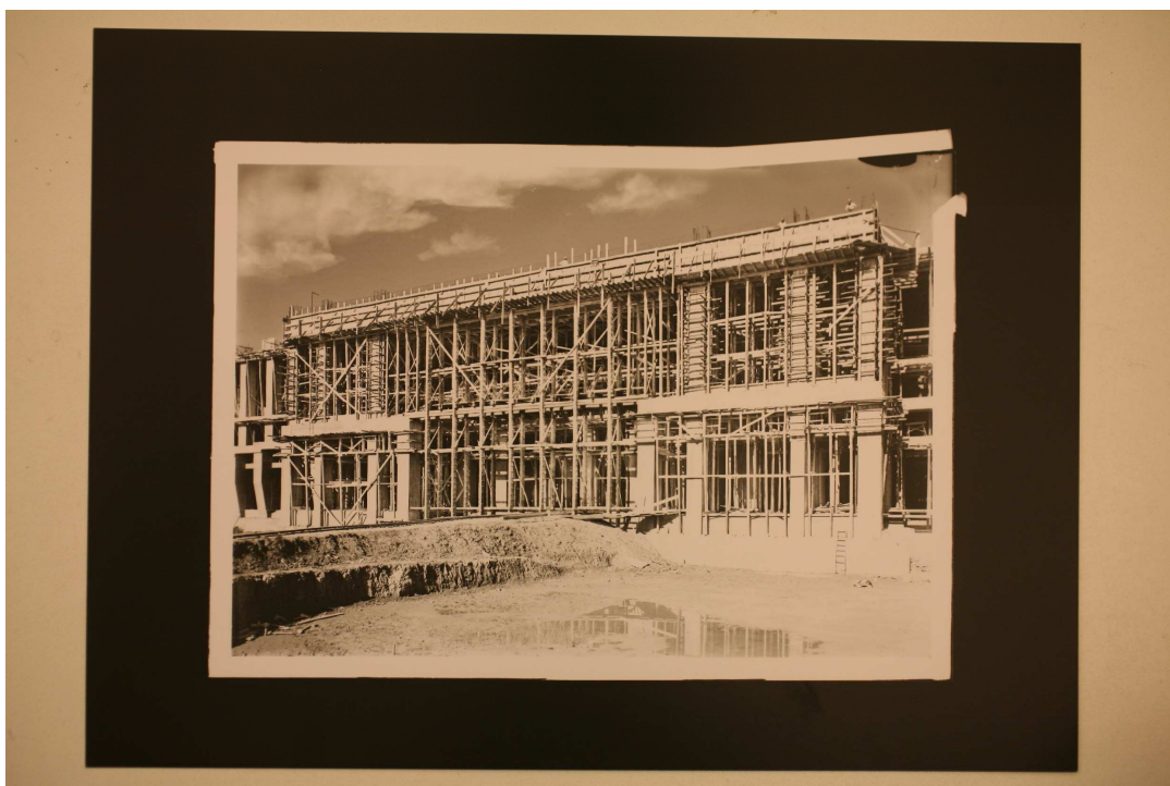
Fig. 104, Archivio Vasari, (Cantiere Palazzo della Farnesina), 1942 c.a., CSAC, sezione fotografia.
