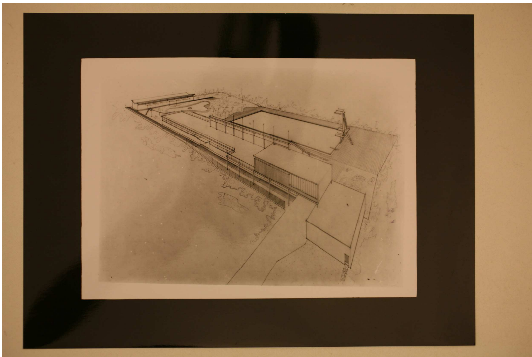
Fig. 126, Archivio Vasari, (Progetto di piscina coperta), 1947, CSAC, sezione fotografia.
